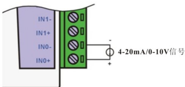
图 4 ISOAD16 模块信号输入接线图
