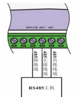
图 3 ISOAD16 模块进入配置状态接线图
