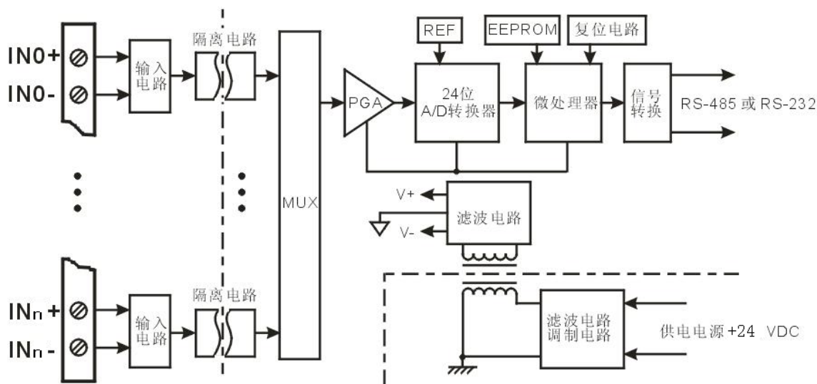
图1 ISOAD 产品原理框图
