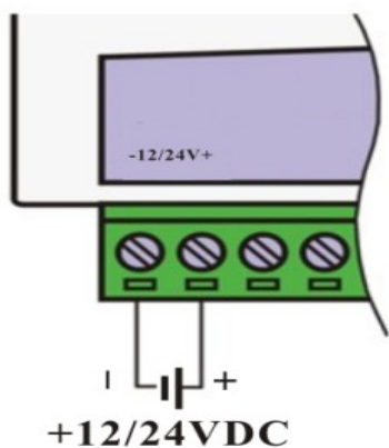
图 2 ISOAD16 模块供电电源接线图
