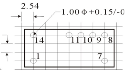
DIP 14 封装
